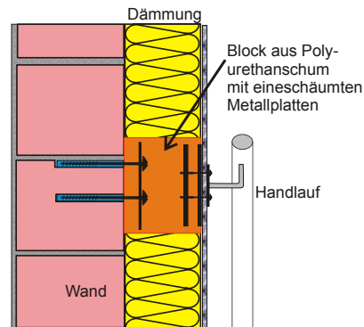
Wärmebrückenarme Befestigung an einer gedämmten Außenwand
