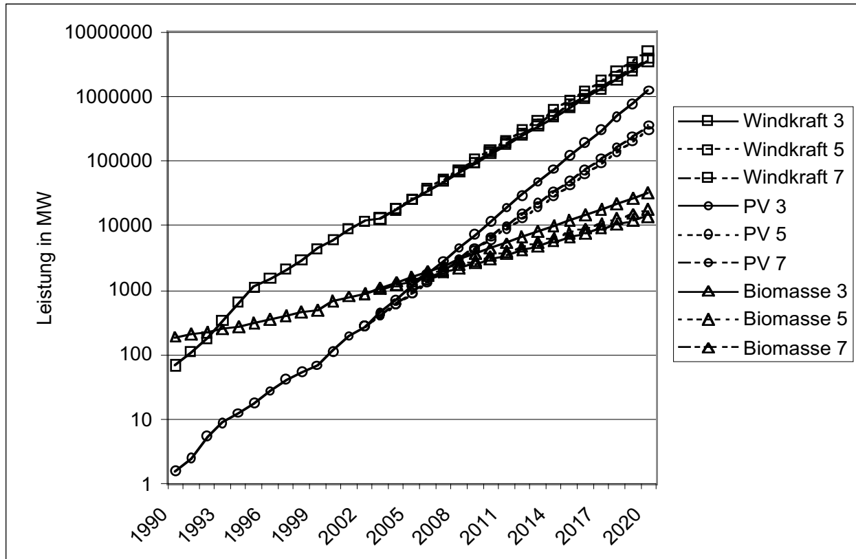
Abb. 1-15 :Fortschreibung des mittleren Wachstums der letzten 3, 5, und 7 Jahre der Entwicklung bis 2020. [eigene Berechnung].
