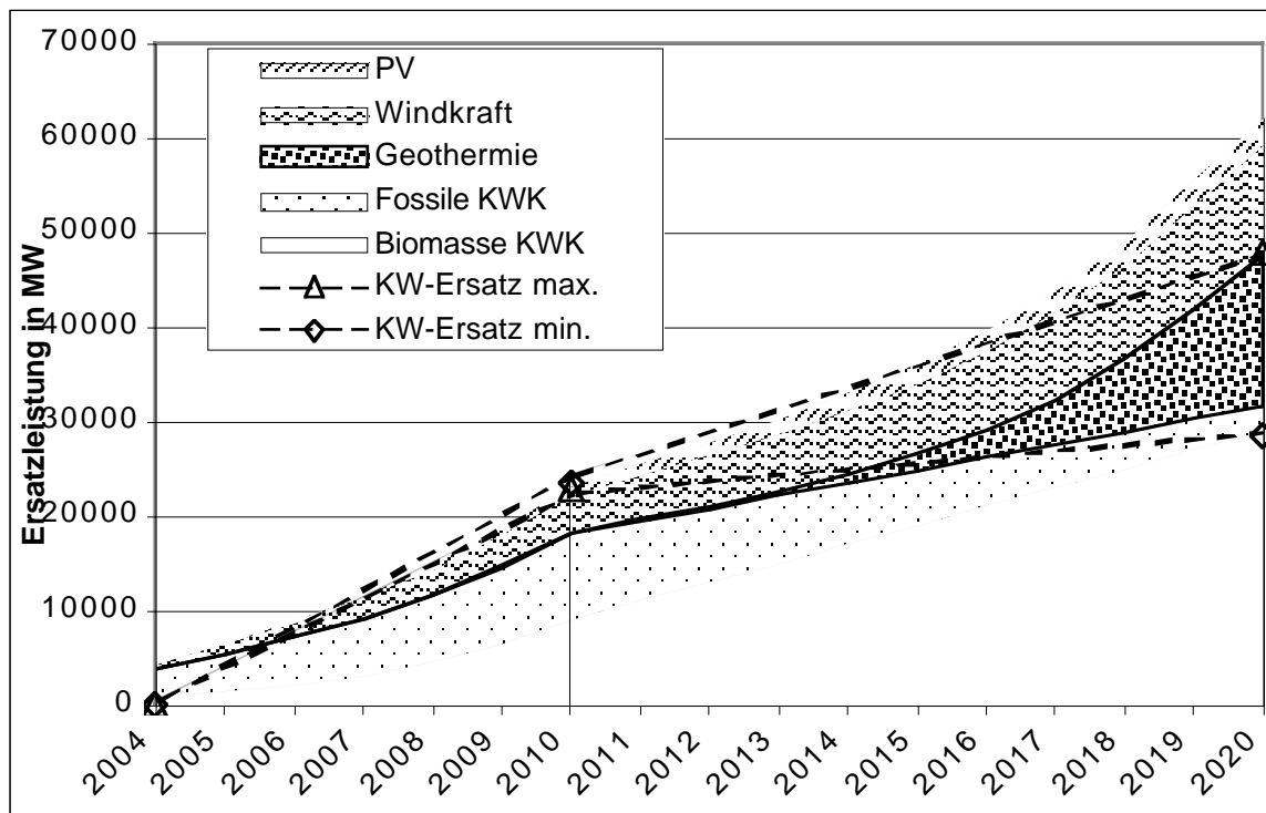
Abb. 1-23 : Erhöhung der durch EE gestellten Kraftwerksersatzkapazität bei einem forcierten Einstieg in die geothermische Stromerzeugung und die Entwicklung der benötigten Kraftwerksersatzleistung unter Berücksichtigung einer Verringerung des Strombedarfs um 1% p.a. durch Effizienzgewinne.
